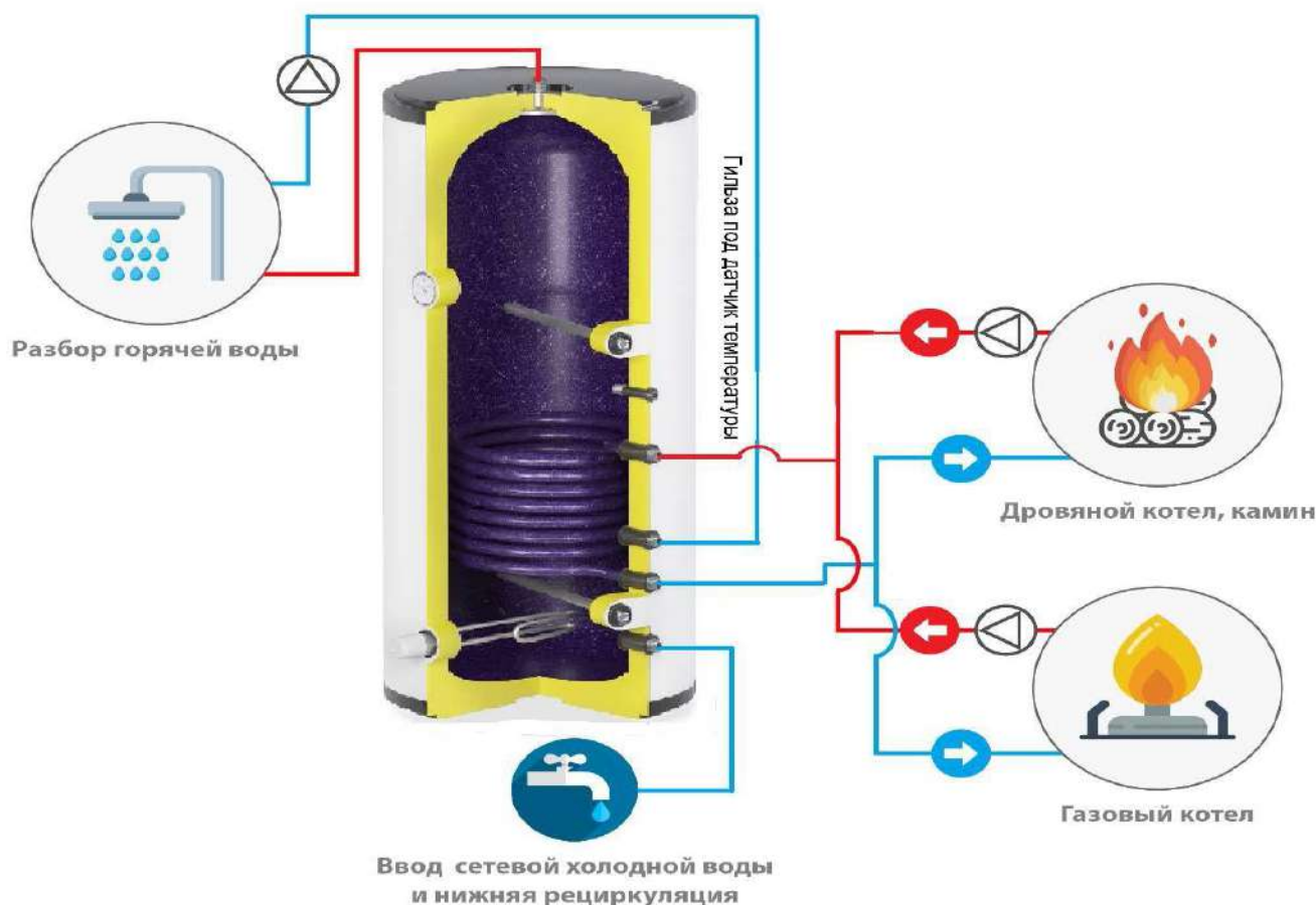
Рис. 1 Гидравлическая схема настенно-напольного водонагревателя STOUT.
