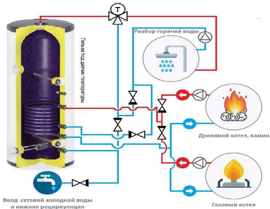
Рис. 2 Гидравлическая схема настенно-напольного водонагревателя STOUT с термостатическим клапаном.
