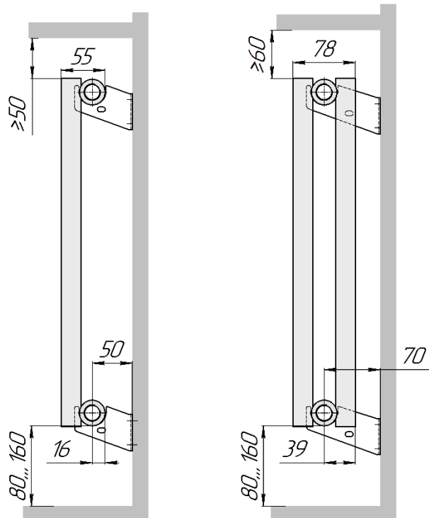
Гармония А25 N 1 (вид сбоку, кронштейны К 50)
