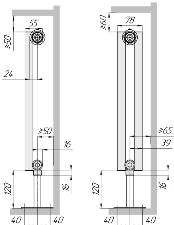
Гармония А25 N 1 нп нв (вид сбоку)
