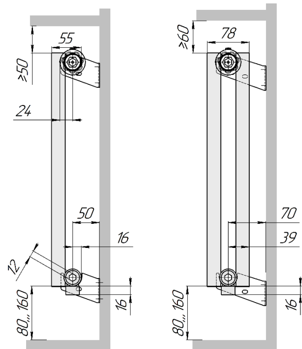
Гармония А25 N 1 нп (вид сбоку, кронштейны К 50)
