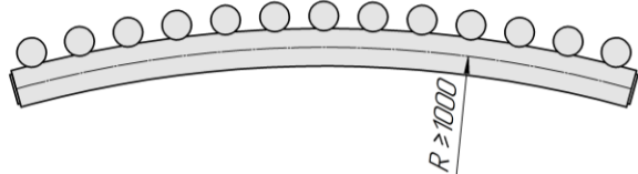
Гармония А 25 N –1 нп R наружн. (вид сверху, изготавливается без встроенного термоклапана)
