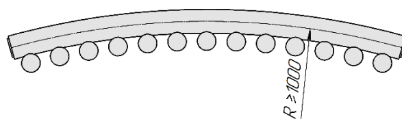
Гармония А 25 N –1 нп R наружн. (вид сверху, изготавливается без встроенного термоклапана)
