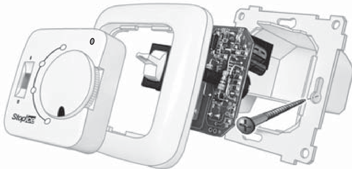
Рис. 3. Сборка терморегулятора
