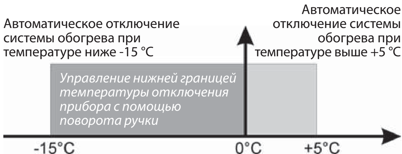
Рис. 2. График работы терморегулятора в зависимости от температуры
