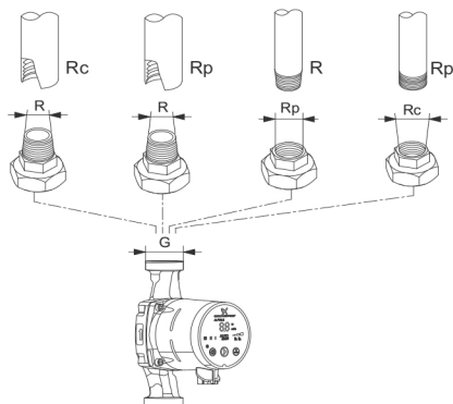
Рис. 23 Резьба G и резьба R
