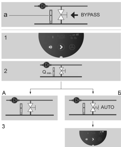
Рис. 18 Системы с перепускным клапаном
