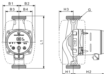
Рис. 19 Габаритный чертёж насосов ALPHA2
