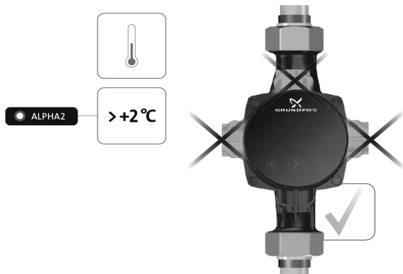
Рис. 7 Допустимое положение головной части насоса при циркуляции холодного теплоносителя
