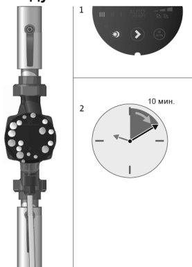
Рис. 11 Удаление воздуха из насоса
