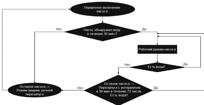
Рис. 16 Алгоритм работы защиты от «сухого» хода
