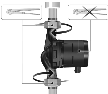
Рис. 4 Затяжка фитингов
