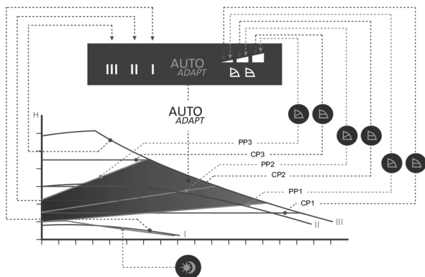
Рис. 14 Расходно-напорная характеристика ALPHA2
