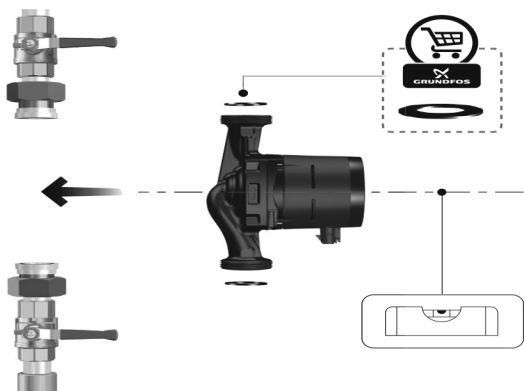
Рис. 3 Монтаж насоса
