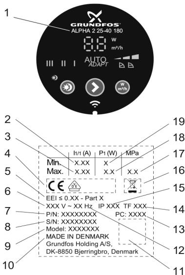
Рис. 1 Фирменная табличка
