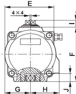
ISO5211 / VDI/VDE3845
