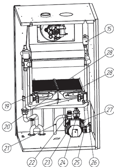
Рис.1. Конструкция котла:
