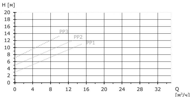
Рис. 8 Кривые режима управления пропорционального изменения давления.
