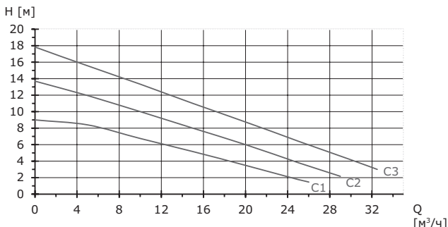
Рис. 10 Кривые режима управления при фиксированной частоте вращения.
