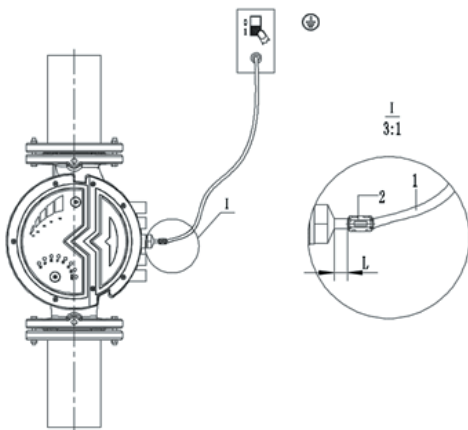
Рис. 6 Электроподключение
