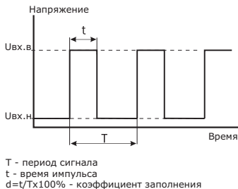
Рис. 11 Характеристики ШИМ-сигнала
