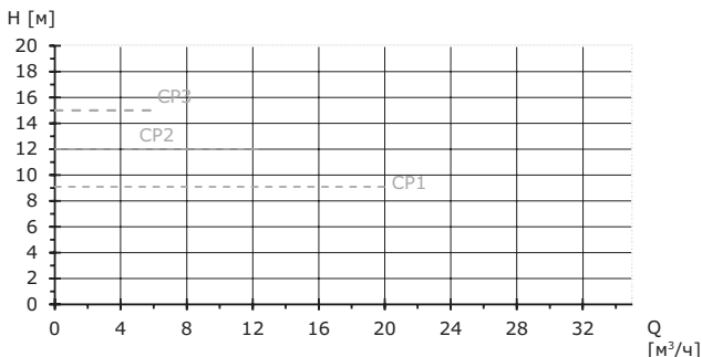
Рис. 9 Кривые режима управления с постоянным значением давления.
