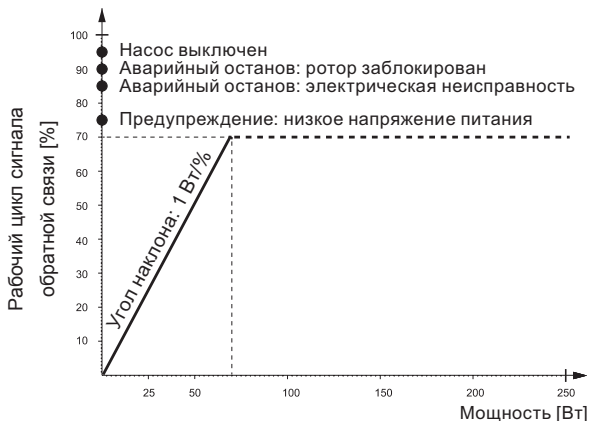
Рис. 13 Зависимость коэффициента заполнения от состояния насоса
